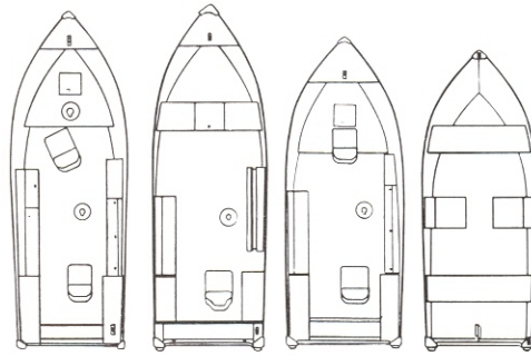
LV16 LTD
